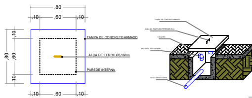
PLANTA BAIXA ESCALA: 1:25
