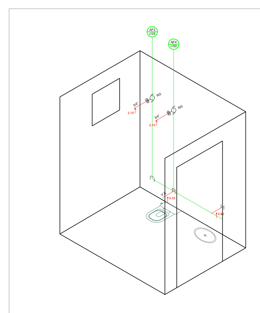
ISOMÉTRICO 01 ESCALA: 1:25
